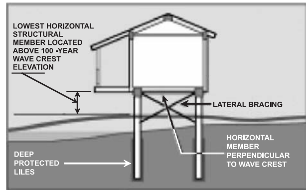
सूनामी प्रभाव से बचने के लिए भवन डिजायन समाधान
